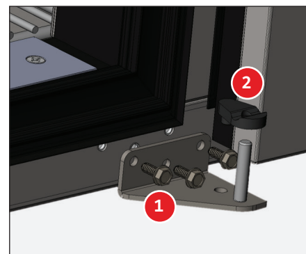
Rys. 9. Zamontować sworzeń zawiasu dolnego w nowym miejscu.
