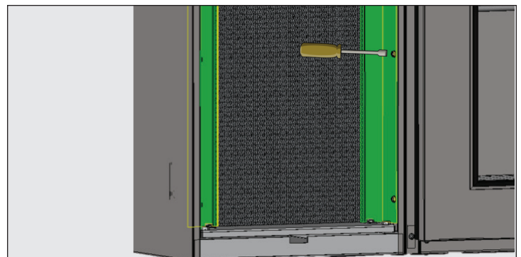
Rys. 6. Zdjąć wsporniki węzownicy.
