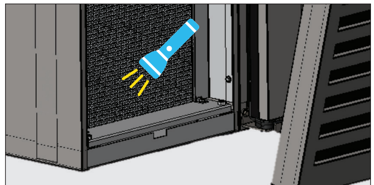
Rys. 4. Sprawdzić, czy wszystkie zatory zostały usunięte.
