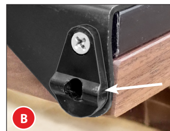
Rys. 5. Zdjąć sworzeń zawiasu górnego i tuleję (A) oraz prowadnicę krzywki drzwi (B) ze wsporników zawiasów. Nie zdejmować wsporników zawiasów.
