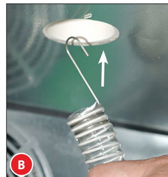
Rys. 7. Przeprowadzenie węża powietrza przez wieżę nalewaka od dołu.
