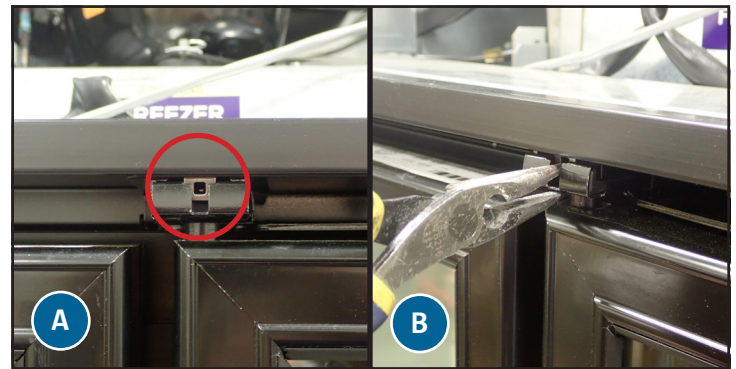
Fig. 6. Goupille de charnière sur le haut de la porte (A). Compression de la goupille de charnière (B).
