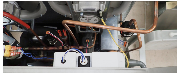
Abb. 2. Draufsicht des TRUEZONE UV-Systems.
