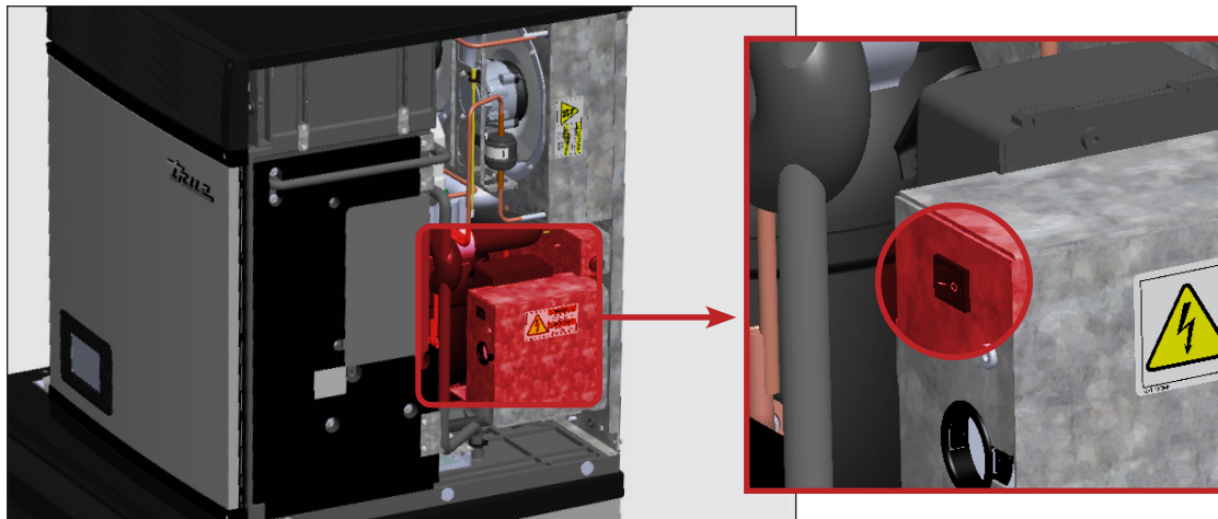
Rys. 2. Położenie przełącznika kołkowego. Przełącznik kołkowy odłącza zasilanie tablicy sterowania i wyświetlacza przedniego, lecz NIE ODŁĄCZA zasilania całego urządzenia.
