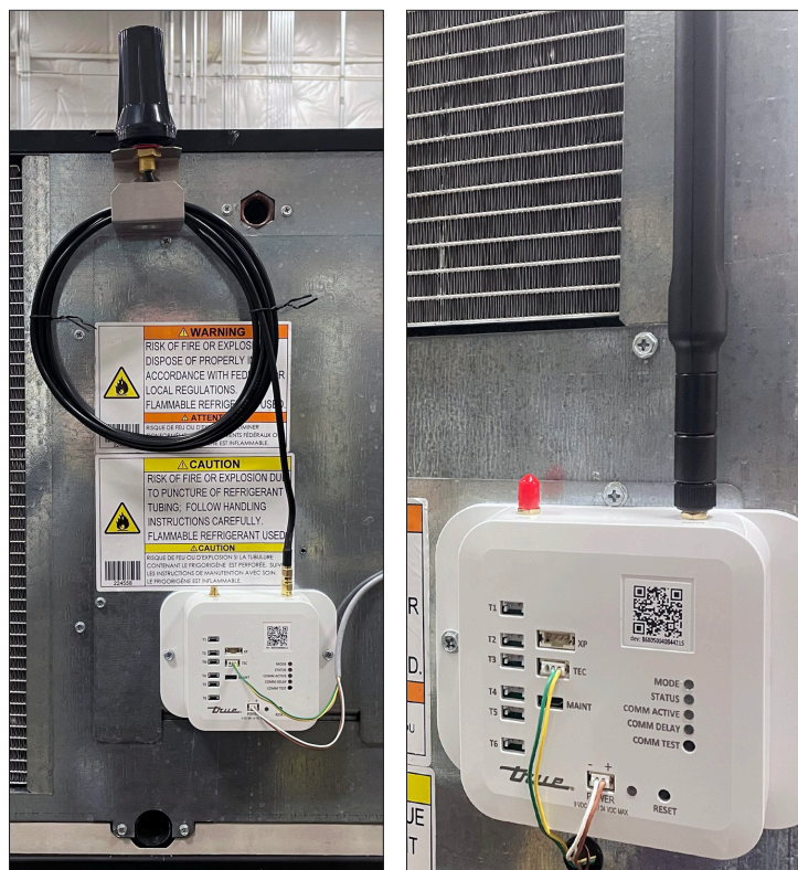
Rys. 3. Zainstalowana na modemie antena. Antena może w rzeczywistości być nieco inna.
