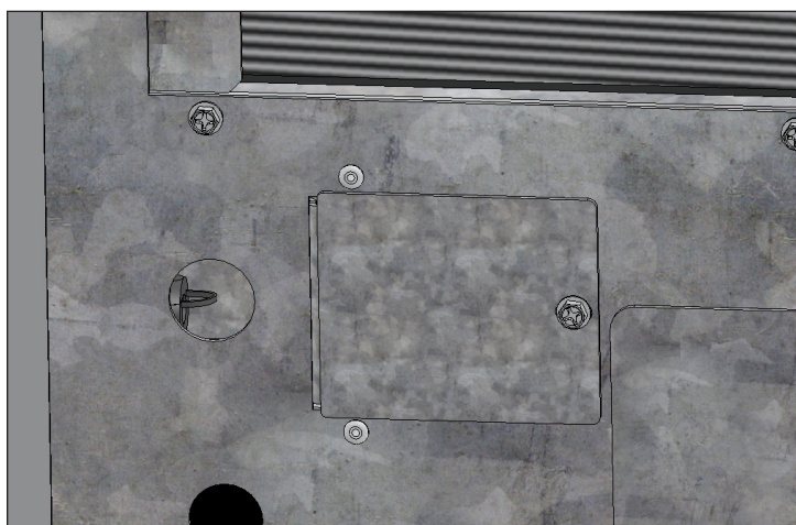
Rys. 2. Położenie przełącznika kołkowego. Przełącznik kołkowy odłącza zasilanie tablicy sterowania i wyświetlacza przedniego, lecz NIE ODŁĄCZA zasilania całego urządzenia.
