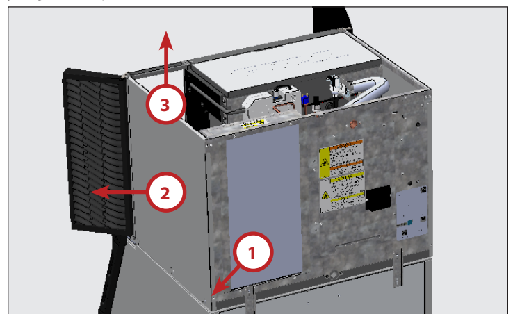
Fig. 3. Quite el tornillo, retire el panel de las pestañas adhesivas y luego levántelo para retirarlo.
