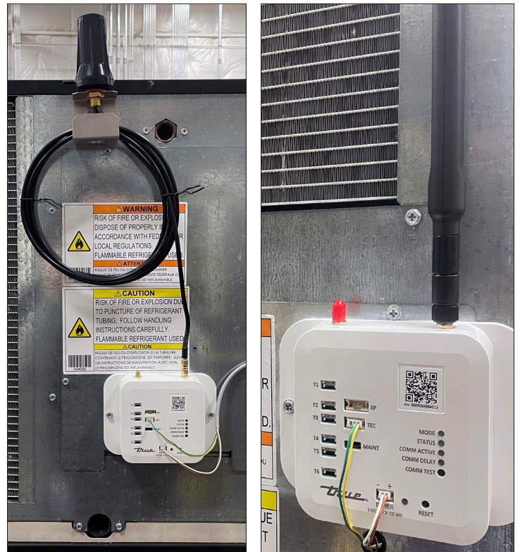
Fig. 3. Antena instalada en el módem. Su antena puede variar.
