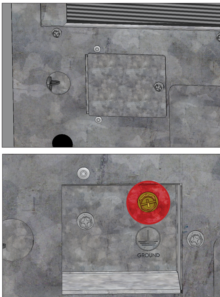
Fig. 3. Realice las conexiones eléctricas dentro de la caja de uniones de la máquina de hielo. Asegúrese de utilizar prensacables. Emplee siempre el tornillo de conexión a tierra de color verde al efectuar conexiones eléctricas.
