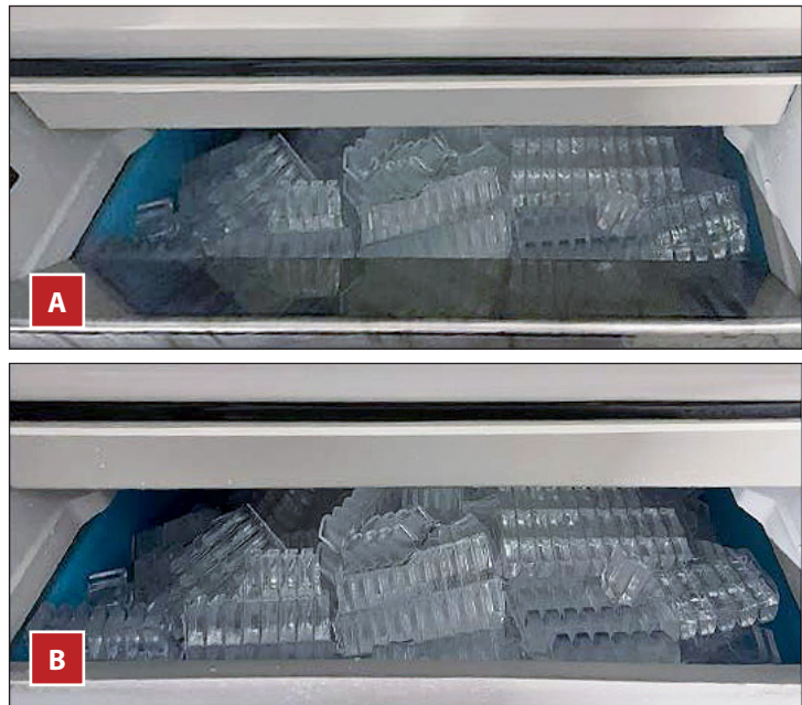
Fig. 5. Depósitos de hielo con (A) y sin (B) deflector de zona de caída.
