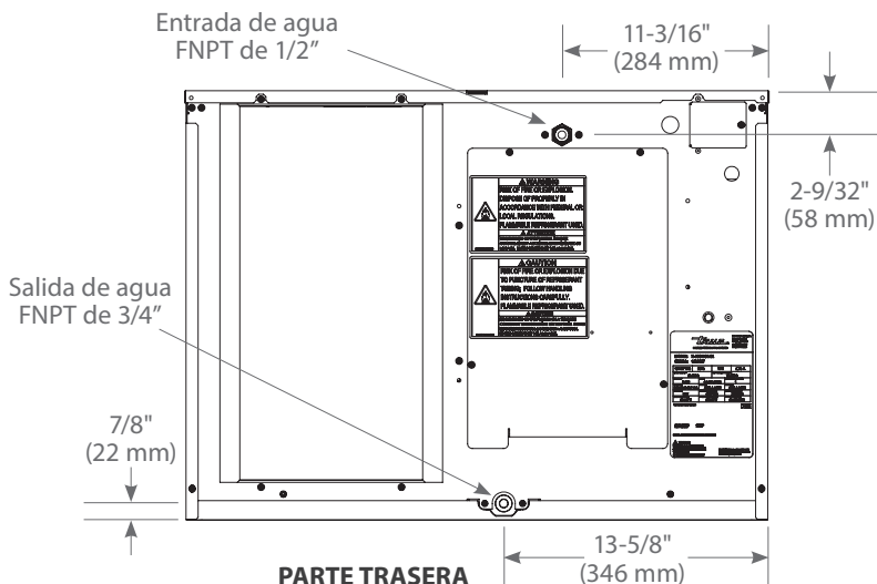
PARTE TRASERA
