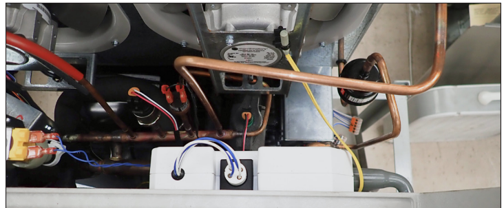
Fig. 2. Vista superior del sistema de luz ultravioleta de TrueZone.
