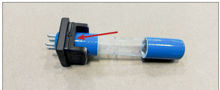
Fig. 4. Muesca del sello de goma.
