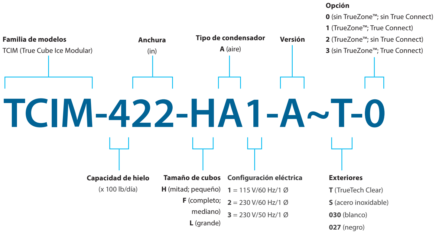
Fig. 1. Diagrama de nomenclatura del modelo TCIM.
