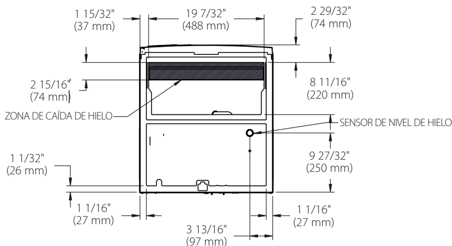
PARTE INFERIOR
