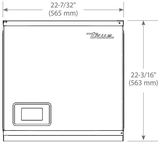
PARTE DELANTERA
