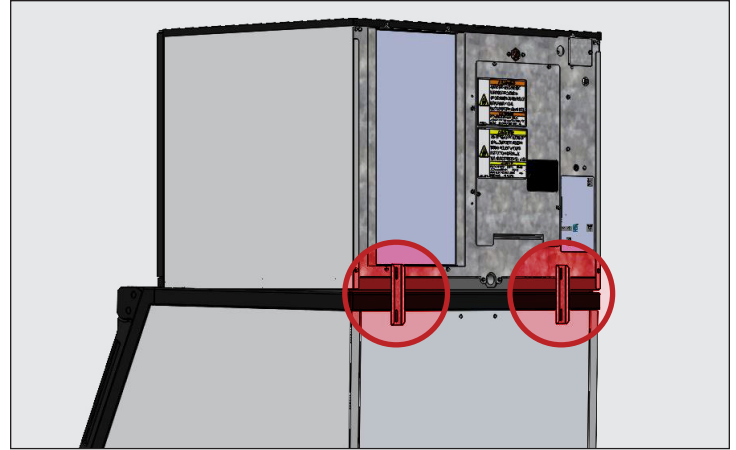
Fig. 1. Soportes del depósito instalados.
