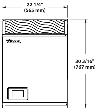
PARTE DELANTERA
