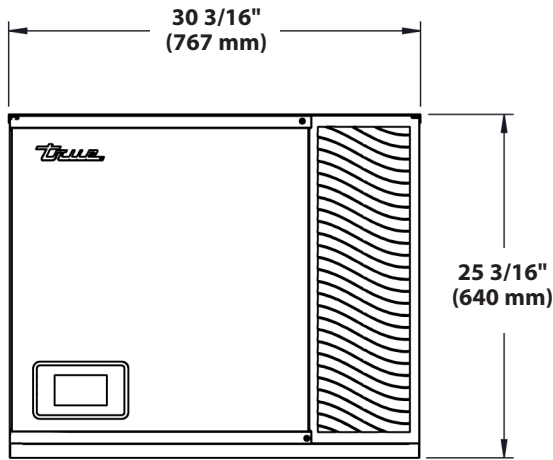
PARTE DELANTERA
