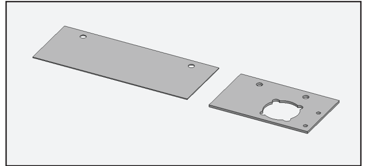
Fig. 16. Placa de cubierta y placa maestra de torsión. Se encuentran en el embalaje interior con las herramientas de nivelación.
