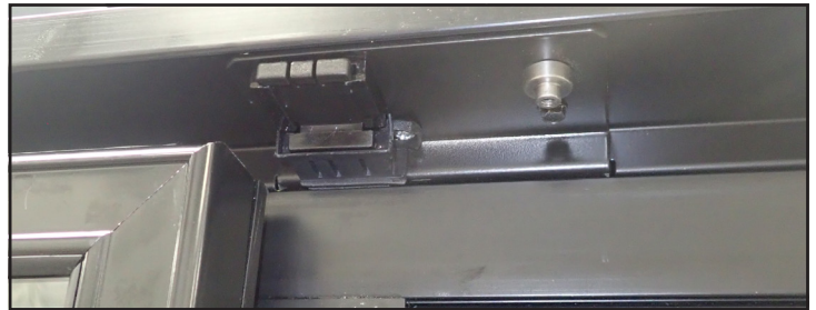
Fig. 23. Tapa del pasador de la bisagra instalado en el lado opuesto.
