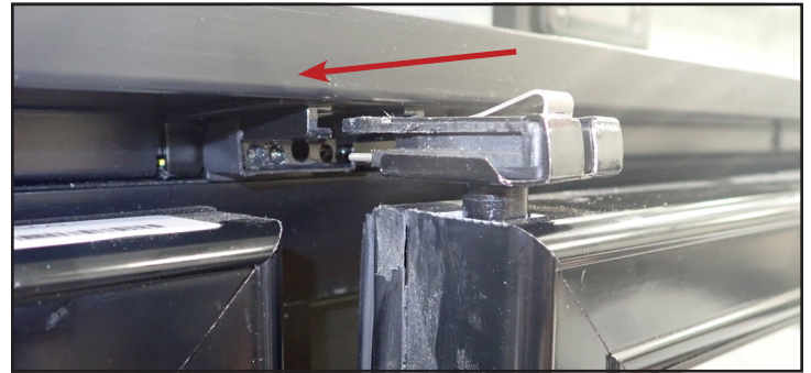
Fig. 9. Alinee el pasador de bisagra.
