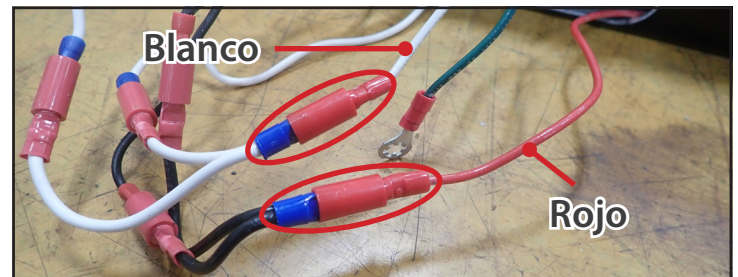
Fig. 19. Conectores de los cables del pasador de bisagra. Estilo n° 1.
