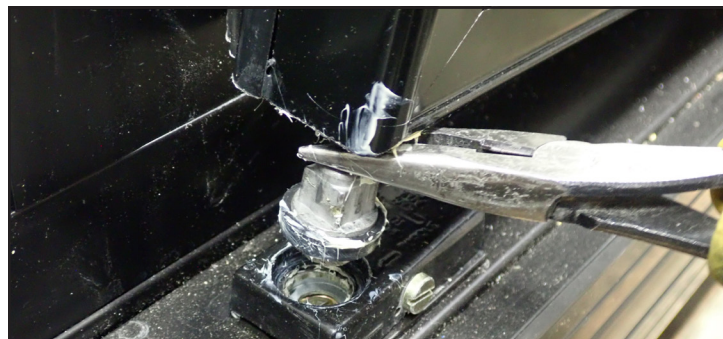
Fig. 8. Un assistant soulevant la tige de torsion du trou du dispositif de réglage de la fermeture de porte (torque master) pendant que le technicien soulève la porte.
