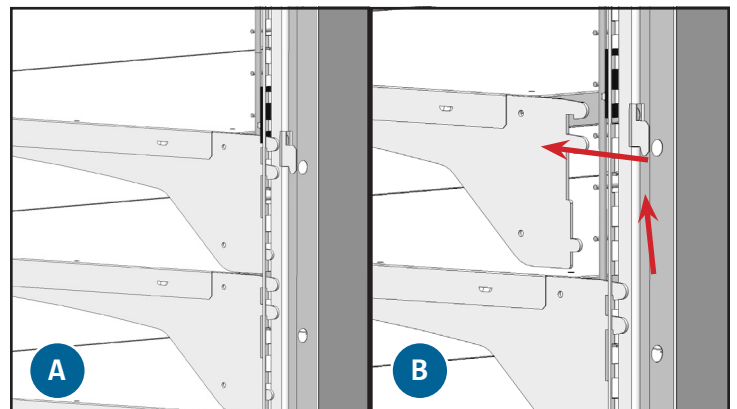
Fig. 4. Soulevez l'étagère et tirez vers l'avant.
