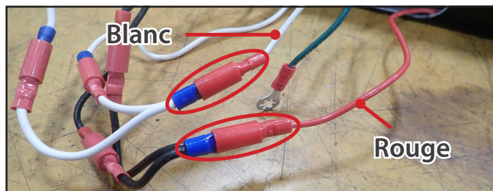
Fig. 19. Connecteurs de câbles de l'axe de charnière. Style #1.
