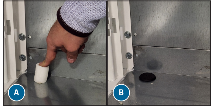
Fig. 1. Boucher (A) un trou des pieds de mise de niveau et le couvrir d'un capuchon (B).
