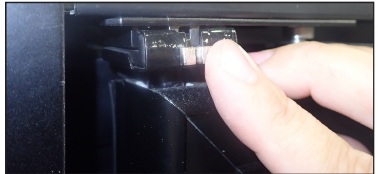
Fig. 12. Insérez le clip de maintien de la charnière.
