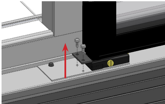
Fig. 1. Retirez la plaque d'expédition de la porte.
