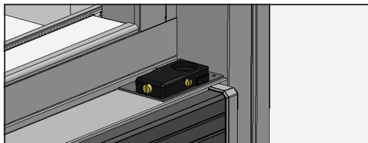
Fig. 27. Ensemble de réglage de la fermeture de porte (torque master) posé correctement.
