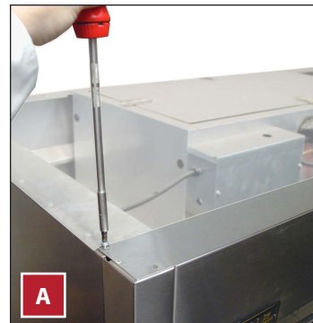
Afb. 3. Verwijder de afdekplaat.
