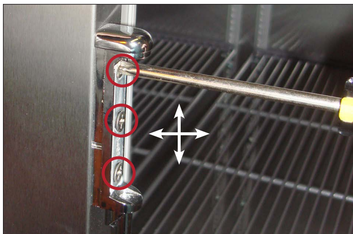
Afb. 4. Locaties schroeven deurscharnier. Stel de scharnier omhoog, omlaag of zijwaarts af.
