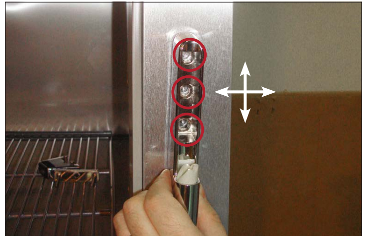
Afb. 2. Locaties schroeven bodemplaat van het scharnier. Stel omhoog, omlaag of zijwaarts af.
