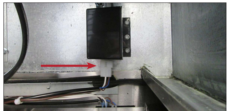
Afb. 4. Ontkoppel de elektronische temperatuurregeling.
