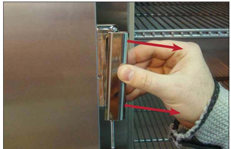
Afb. 3. Trek de scharnierplaat van de deurscharnieren.
