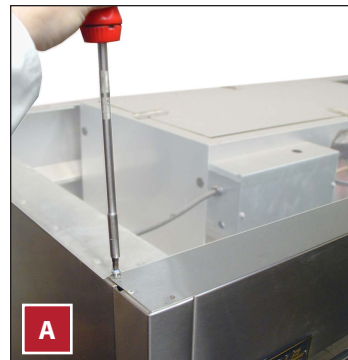
Abb. 3. Regenabweiser entfernen.
