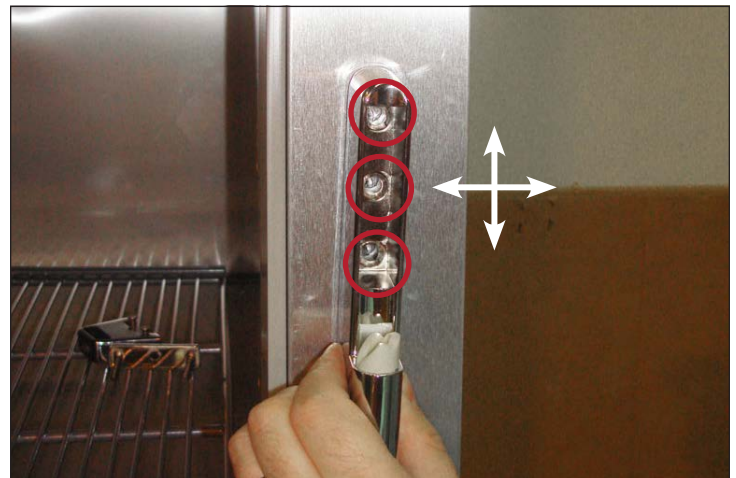
Fig. 2. Ubicación de los tornillos de la base de la bisagra. Ajuste hacia arriba, hacia abajo o lateralmente.
