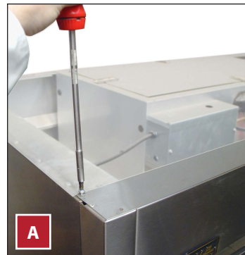
Fig. 3. Retire el protector para lluvia.
