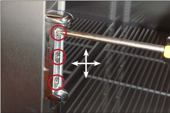
Fig. 4. Ubicación de los tornillos de las bisagras de la puerta. Ajuste la bisagra hacia arriba, hacia abajo o lateralmente.
